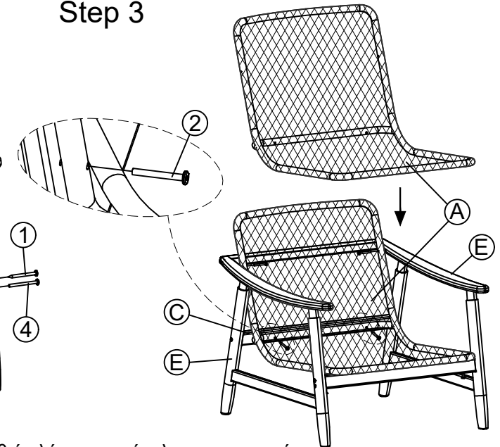
④ Bolt M6 x 70 = 4 pcs
